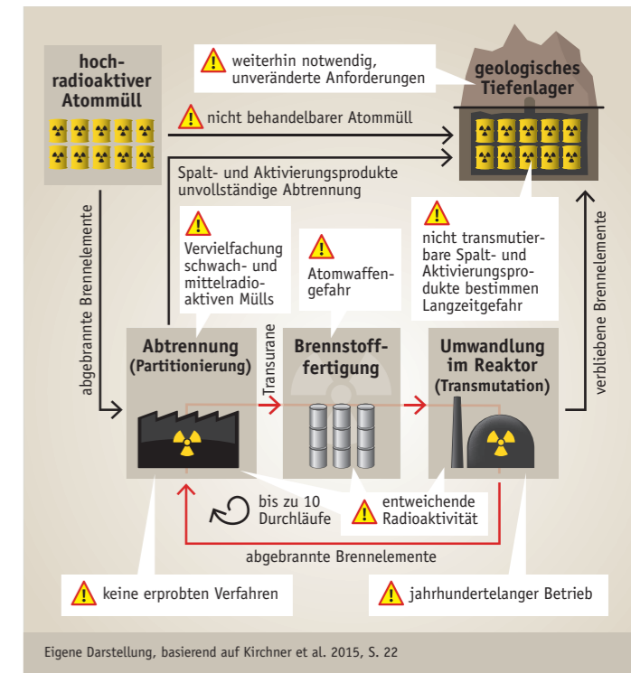
Schematische Darstellung der Transmutations-Idee und ihrer Probleme
