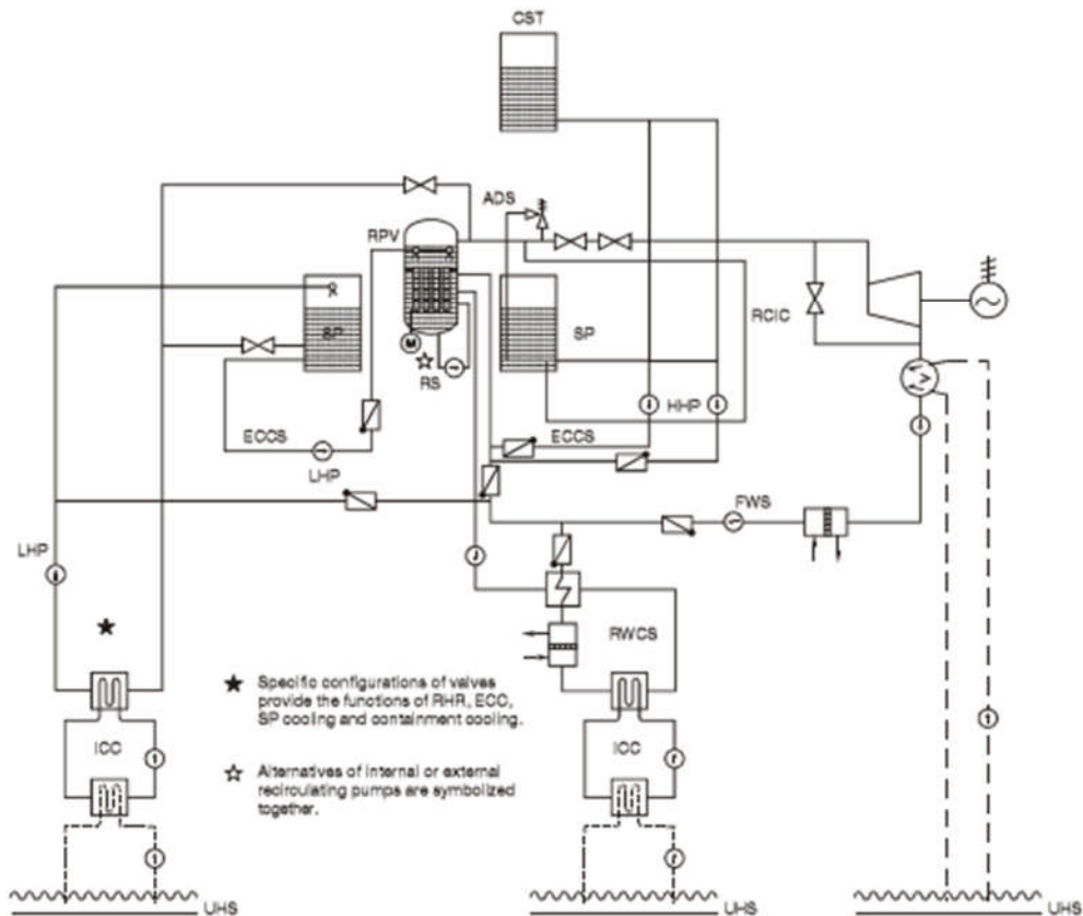
Bild 8: Empfehlungen der IAEA zum Aufbau eines Not- und Nachkühlsystems für einen Siedewasserreaktor (SWR) /31/
